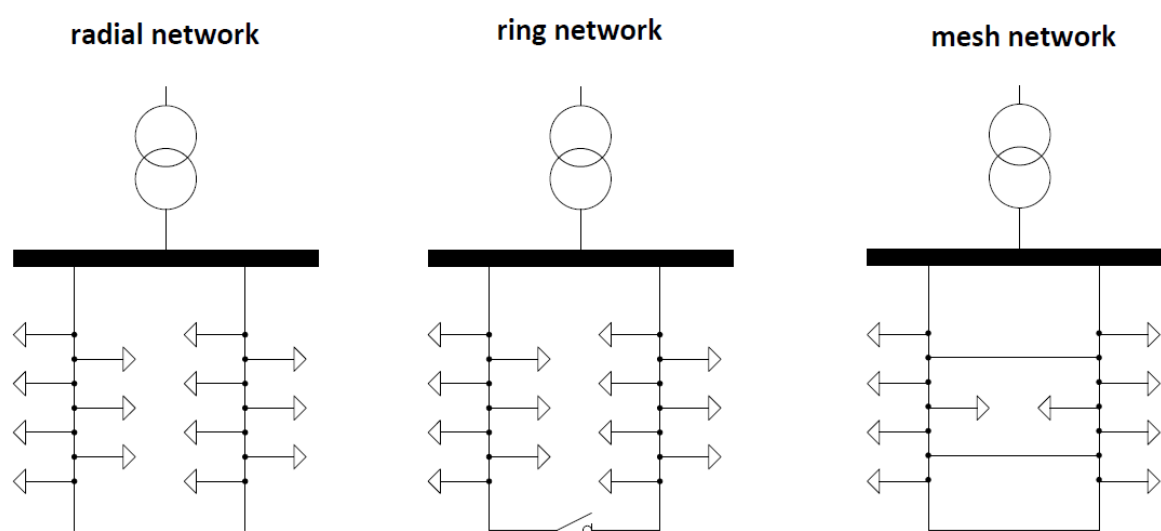
Figure 39: Overview of different network typologies based upon, Source: (Aufnahmefähigkeit von Niederspannungsverteilnetzen für die Einspeisung aus Photovoltaikanlagen, 2011)
